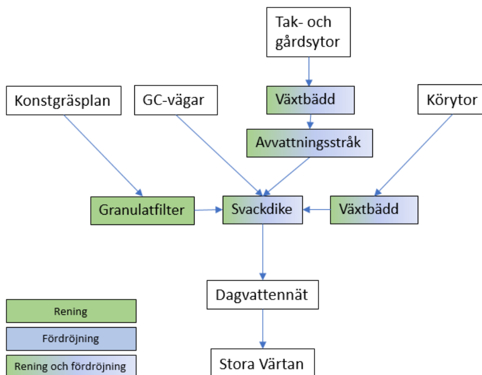
Figur 12 Schematisk skiss över föreslagen dagvattenhantering. Färgerna anger rening och-/eller fördröjning.
